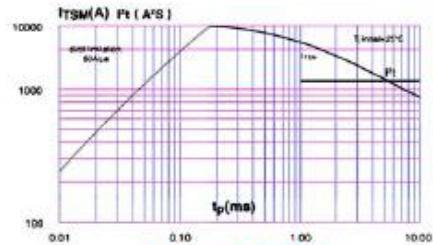
6、 I_{TSM}-t, Ft-t 曲线
