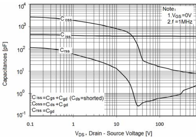
Figure10. Capacitanc
