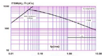
6、 I_{TSM}-t, I_T^2-t 曲线
